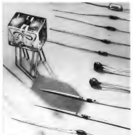
Bild 8. Elektronische Baugruppe in Siemens-Mikroblock-Bauweise. Auf kleinstem Raum ( 10\text{ mm} \times 8\text{ mm} \times 6,3\text{ mm} ) bilden fünfzehn konventionelle Kleinbauelemente, wie sie rechts liegen, einen bistabilen Multivibrator
