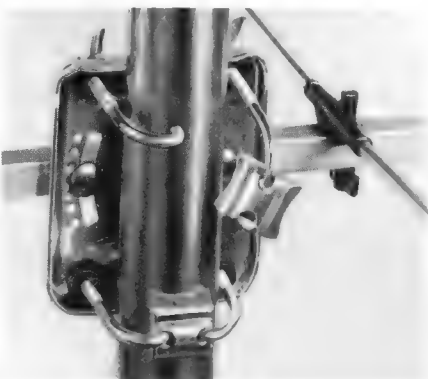
Bild 8. Die Mastschelle ist unterteilt; die beiden Hälften werden bei der Montage in das Verbindungsstück eingehakt, so daß die Flügelmutter nicht mehr ganz abgeschraubt werden müssen (Zehnder)
