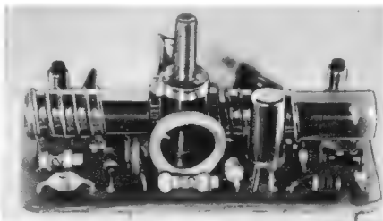
Bild 8. UKW-Variometer 1755 von Vogt & Co. Der Baustein ist mit zwei Transistoren bestückt, der Abstimmkern verschiebt sich zügig und spielfrei in dem Spulenrotor mit der Vorkreis- und Oszillatormwicklung (Vogt & Co.)
