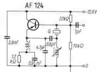
Bild 18. 27,5-MHz-Oszillator hoher Frequenzkonstanz mit Steuerquarz Q (Valvo)
