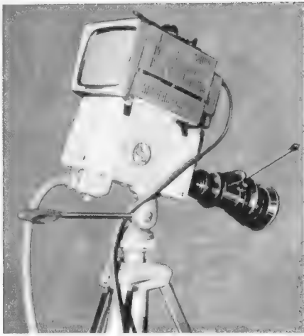
Bild 3. Transistor-Fernsehkamera mit Vario-Optik und aufgesetztem japanischen Kleinfernsehgerät als elektronischer Sucher (Kamera: Fernseh GmbH), zusammengestellt von Loewe-Opta für den Videoaufzeichnungs-Vorführwagen
