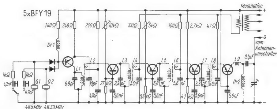
Bild 8. Schaltung des Senderteiles eines volltransistorisierten Funksprechgerätes für zwei Kanäle (145 und 145,5 MHz) von SEL
