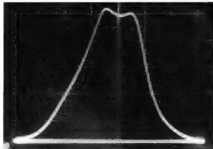
Bild 8. Normale Durchlaßkurve eines Tuners. Die Marke für die Mittenfrequenz 36,15 MHz deckt sich mit der Skalenmitte
