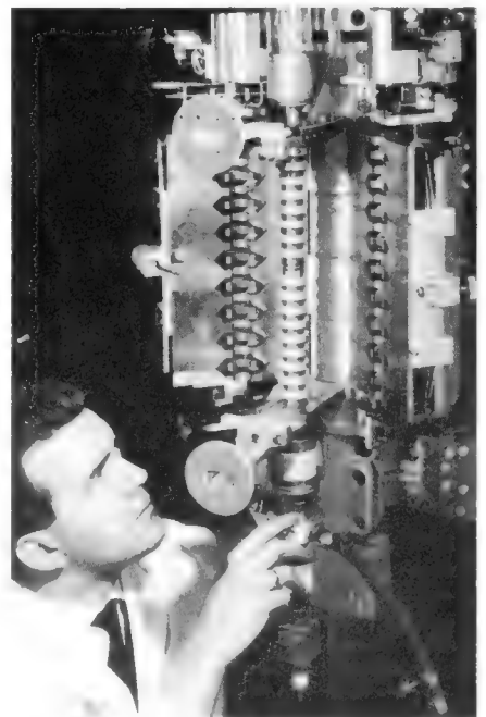
Bild 2. Siemens-Hochleistungs-Wanderfeldröhre YH 1040 mit aufgeklapptem Magnetsystem; die Röhre ist für interkontinentale Nachrichtenverbindungen über künstliche Satelliten bestimmt
