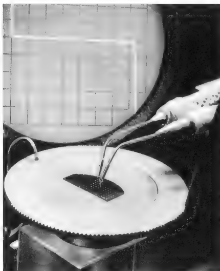
Bild 2. Vergrößerter Ausschnitt einer Meßanordnung für Planartransistoren; die Kennlinie ist auf dem Schirm sichtbar (Siemens)
