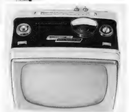
Unten: Bild 2. Transistor-Fernsehgerät Astronaut Modell 1514 (Kuba/Imperial) mit Feldstärke-meßgerät für Antennenmontage
