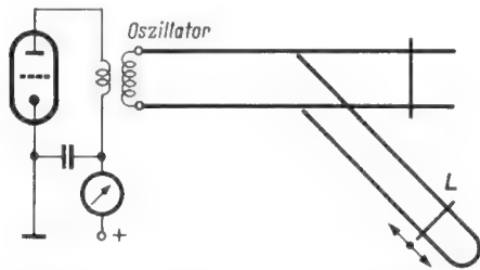
Bild 1. Frequenzbestimmung mit einem lose angekoppelten, in seiner Länge veränderlichen Leitungskreis; L = veränderlicher Leitungskreis
