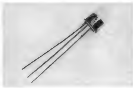
Bild 22. Ditratherm-Halbleiter; links = Video-Endstufentransistor BF 108, rechts = Silizium-Boosterdiode Typ SFR 105 A für Fernsehempfänger
