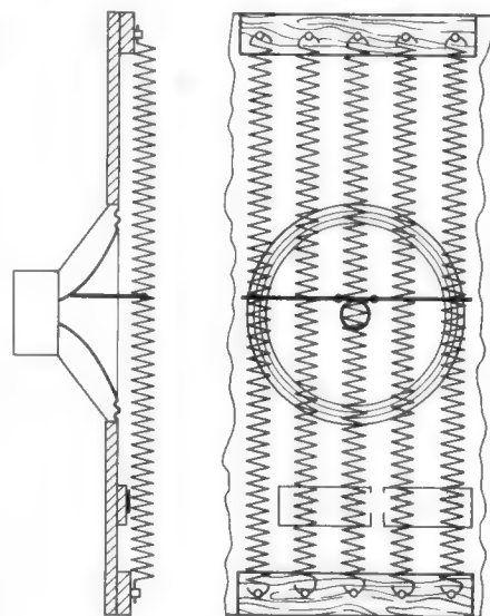
Bild 11. Audax-Nachhall-Lautsprecher (Frontansicht)
