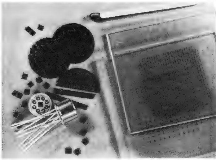
Bild 4a. Montierter und kontaktierter Festkörper-Schaltkreis auf dem Sockel eines TO-5-Gehäuses (Valvo)
