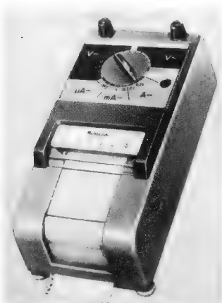
Bild 1. Vielfachinstrument Multiscript 3 mit eingebautem Schreiber (Metrawatt)
