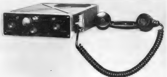
Bild 1. Teleport VI (rechts Batterie, links Nf-Zusatz mit 0,5-W-Verstärker und Mikrofon/Lautsprecher)
