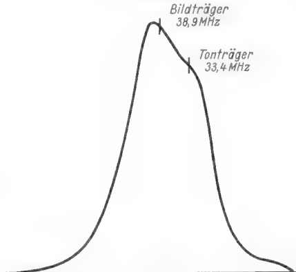
Bild 10. Verformte Durchlaßkurve bei Ankopplung des Tastkopfes über einen Kondensator von 1 nF
