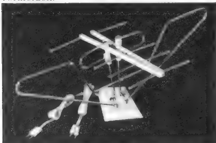
Bild 9. Kombinations-Zimmerantenne für die VHF- und UHF-Bereiche. Beide Einzelantennen werden über getrennte Zuleitungen mit dem Empfänger verbunden (Zehnder)
