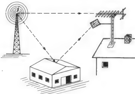
Ein vereistes Dach reflektierte das Fernsehsignal zusätzlich schräg von unten in die Antenne. Eine selbstgebaute Abschirmwand aus Kupfergeflecht beseitigte das Geisterbild
