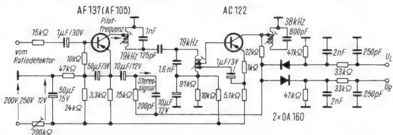
Bild 15. Stereo-Adapter nach Telefonen; der Transistor AC 122 arbeitet als 19-kHz-Oszillator und Frequenzverdoppler, um den 38-kHz-Hilfsträger zu erzeugen
