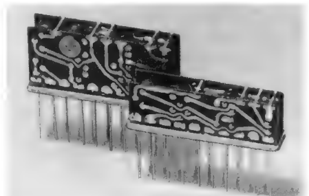
Bild 9. Valvo-Digital-Baustein vor dem Vergießen, ohne Gehäuse
