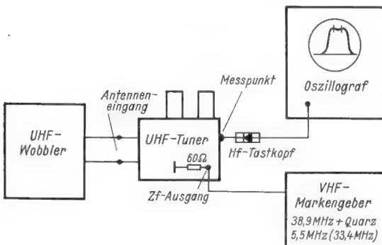
Links: Bild 13. Aufbau des UHF-Meßplatzes. Wenn der VHF-Markengeber einen 60-Ω-Ausgang besitzt, kann der Abschlußwiderstand am Zf-Ausgang des Tuners entfallen
