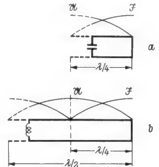
Bild 3. „Leistungsverkürzung“ und „Leistungsverlängerung“; a = Verkür-zung einer \lambda/4 -Leitung; b = Verkür-zung einer \lambda/2 -Leitung oder Verlän-gerung einer \lambda/4 -Leitung
