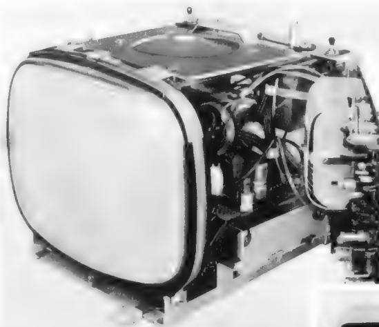
Links: Bild 1. Transistor-Fernsehgerät Transvisa (Nordmende) mit 25-cm-Bildröhre. Man erkennt die herausgeklappten, durch Stecker verbundenen Chassisteile
