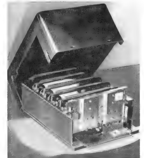
Bild 5. Gehäuse mit fünf Transistor-Verstärkereinsätzen und einem Netzeinsatz. Vorn der UHF-Verstärkereinsatz von Bild 6 (Siemens)
