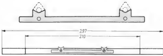
Oben ein beschnittener und gebohrter Leitz-Broschüren-Einhänger, darunter die Leiste mit dem aufgeschraubtem Broschüren-Einhänger und zwei Strichmarken für DIN-A 5-Hefte
