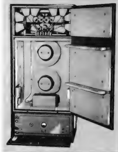
Bild 10. Studio-Abhörschrank O 85 a von Telefunken
