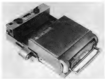
Transistor-Universalempfänger Transmobil in italienischer Form mit der zugehörigen Autohalterung
