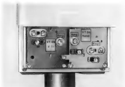
Bild 7. Zwei Transistor-Antennenverstärker für je einen Kanal im Bereich III und IV in einem gemeinsamen Gehäuse zur Montage am Standrohr (Teilansicht; Wisi)
