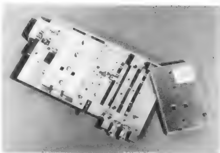
Bild 6. Verstärkereinsatz für einen Kanal im UHF-Bereich. Die hier abgenommene Abschirmkappe schützt außerdem gegen mechanische Beschädigung der Abstimmeelemente (Siemens)
