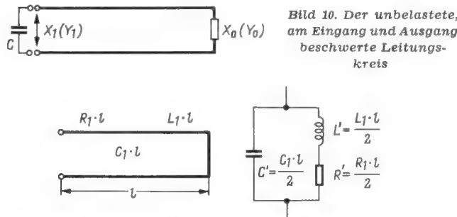
Bild 11. Eine unbeschwerte, nur mit Längsverlusten behaftete (belastete) Leitung, ersetzt durch einen äquivalenten Schwingkreis mit konzentrierten Kreiselementen
