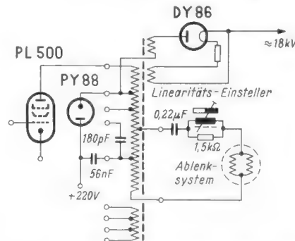
Bild 1. Vereinfachte Darstellung einer Zeilenkippen-Endstufe mit dem Linearitäts-Einsteller
