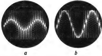
Bild 16. Oszillogramme von Hochfrequenz-Stereosignalen; a = 1-kHz-Signal rechts + 60-Hz-Signal links. Die Amplitude des 60-Hz-Signals ist kleiner; b = 1-kHz-Signal rechts + 60-Hz-Signal links bei gleicher Amplitude
