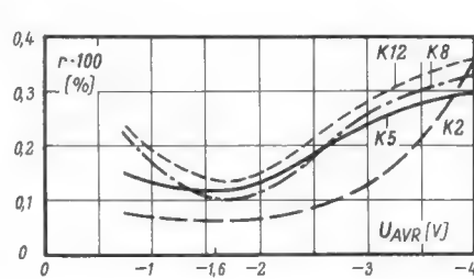
Bild 2. Reflexionsfaktor in Abhängigkeit von der Verstärkungsregelung; K = Kanal
