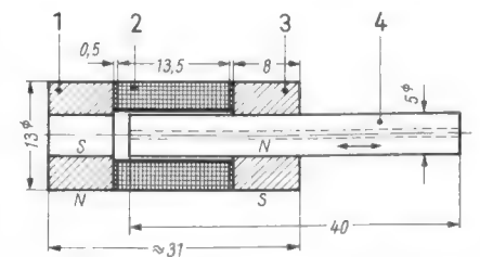
Bild 2. Schnitt durch einen Linearitäts-Einsteller nach SEL-Unterlagen. Es bedeuten: 1 und 3 = gegenseitig gepolte Ferroxdure-Magnete, 2 = Spule aus 147 Windungen 0,5 CuL, 4 = Rohrkern
