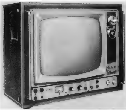
Bild 5. Nordmende-Fernseh-Kontrollempfänger FKE 347
