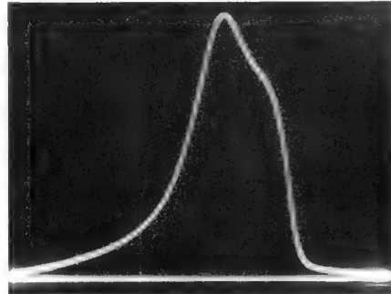
Bild 7. Verzerrete Durchlaßkurve infolge Fehlens des 60- \Omega -Abschlußwiderstandes am Zf-Ausgang
