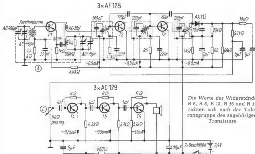
Bild 14. Schaltung eines AM-Taschenempfängers mit Telefonen-Submin-Transistoren
