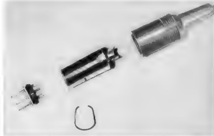
Bild 7. Normstecker für Phono- und Tonbandgeräte; die einzelnen Teile rasten beim Montieren so sicher miteinander ein, daß keine Schrauben notwendig sind (Lumberg)
