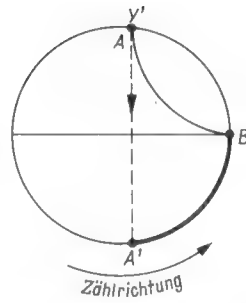
Bild 5. Die kapazitive Beschwerung am Leitungsanfang — dargestellt im Kreisdiagramm (betrachtet vom Leitungsende aus). Punkt A ist gegeben durch den normierten Blindleitwert von C.
