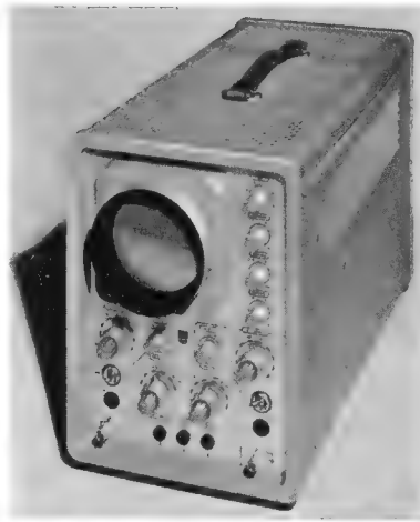
Bild 10. Philips-XY-Oszillograf GM 5639
