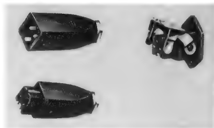
Bild 5. VDE-gemäße Kleinnetzsteckverbindung; links Stecker und Kupplung, rechts Einbaubuchse mit Sicherungsbügel (Hirschmann)
