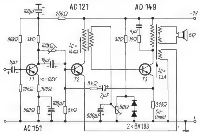
Bild 11. Nf-Verstärker mit 4-W-Eintakt-Endstufe nach Siemens
