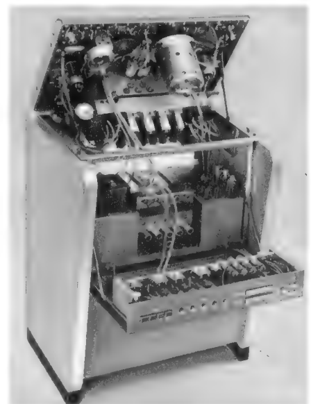
Bild 5. Studio-Magnettongerät J 37 (Franz KG)
