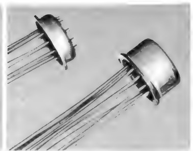
Bild 4b. TO-5-Gehäuse für einen Valvo-Festkörper-Schaltkreis mit zehn Anschlüssen; links der Sockel mit den Elektroden, rechts das geschlossene Gehäuse
