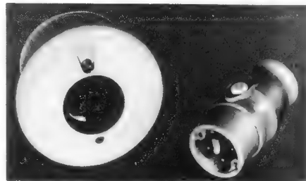
Bild 6. Unterputz-Ausführung der Netzsteckverbindung für Studio und Labor. Die Unverwechselbarkeit sichert phasengleichen Anschluß aller Geräte (Tuchel)
