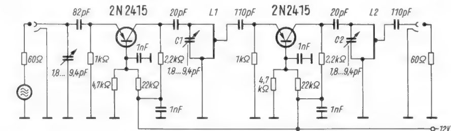
Bild 17. 450-MHz-Verstärker mit Transistoren von Texas-Instruments; L 1 - C 1 und L 2 - C 2 sind durchstimmbare Topfkreise
